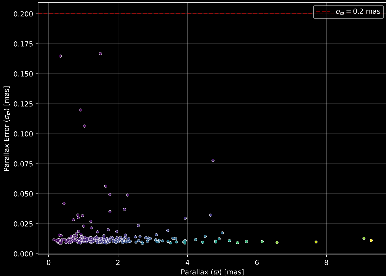
GALAH DR4 Field: [1336] Parallax Quality (n= 272)
