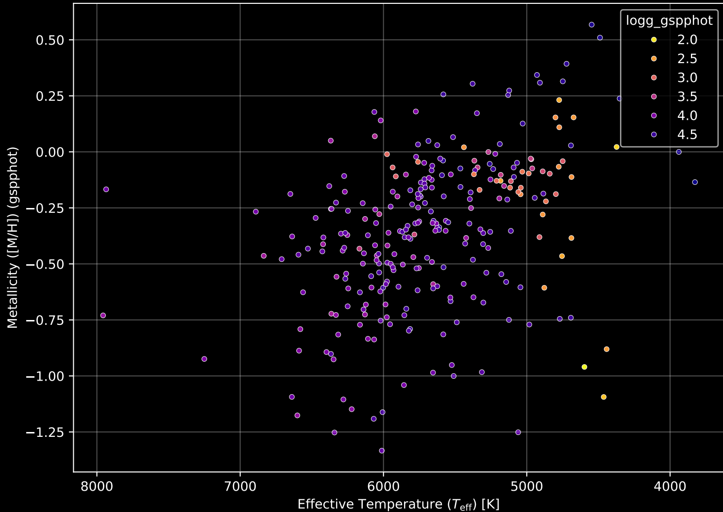
GALAH DR4 Field: [1336] Stellar Population Parameters (n= 272)
