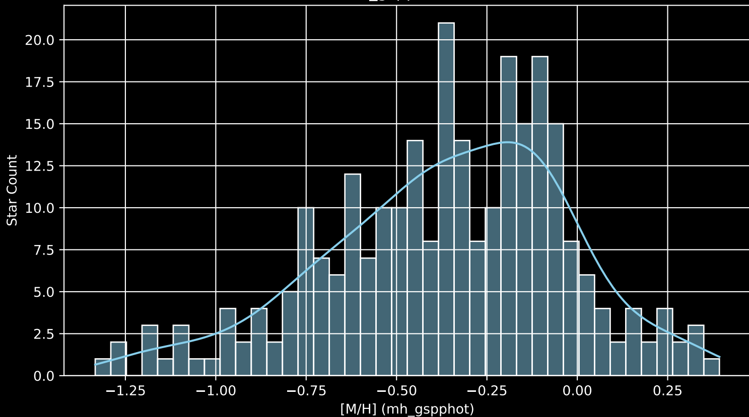
GALAH DR4 Field: [1336] [M/H] (mh_gspphot) (n= 270)
